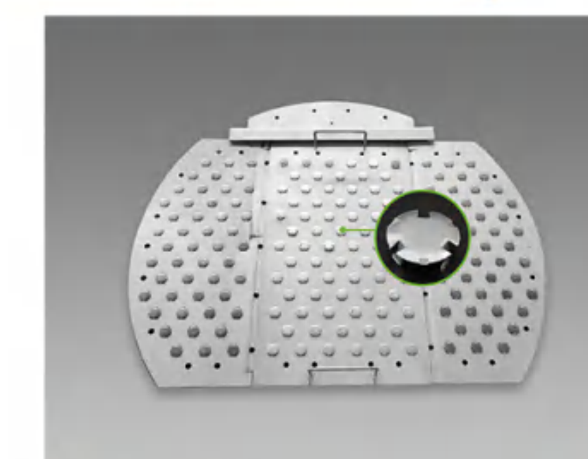
F1 float valve tray
